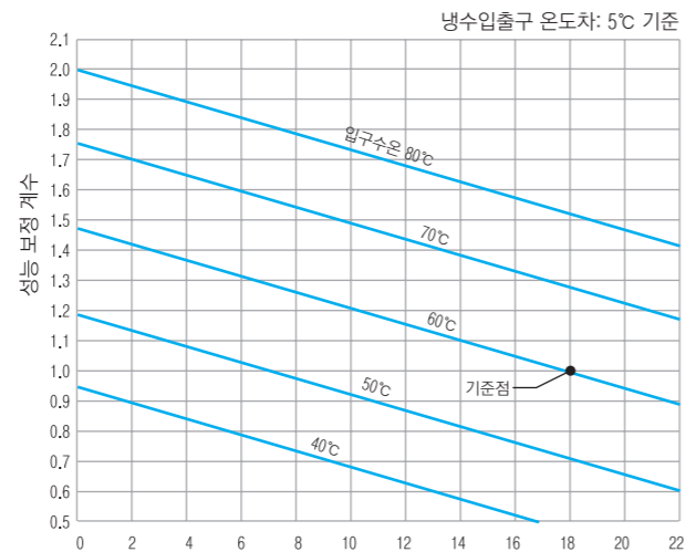
그림 3 5/8"온수코일 용량보정계수(Capacity Correction Factor of Hot Water Coil)
