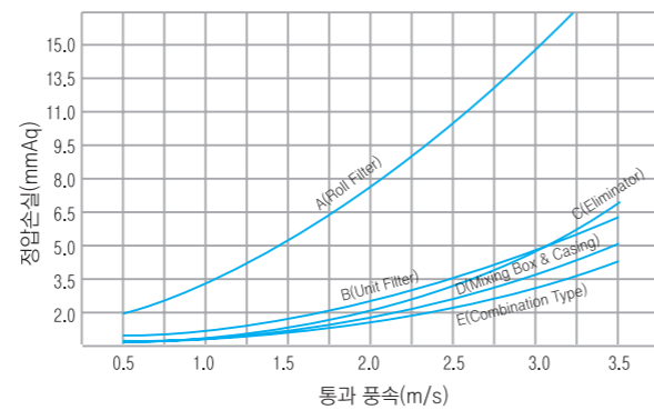
그림 8 에어필터, 엘리미네이터, 믹싱박스 및 케이싱, 복합형 보정 정압손실
