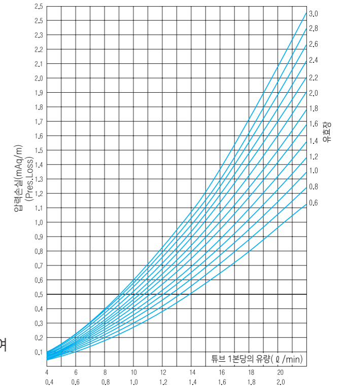
그림 4 냉·온수코일 압력손실(Cold and Hot Water Pressure Loss)
