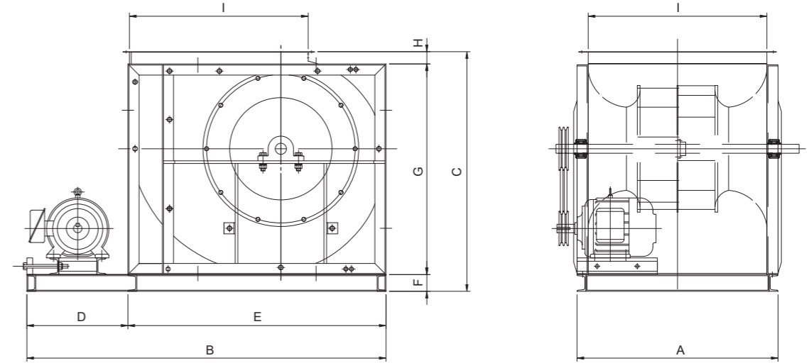
Fan Ass'y Size (AYZ, TYZ)
