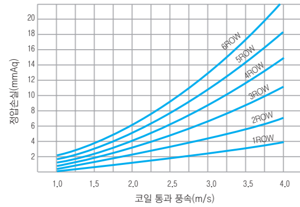
그림 7 온수 및 증기코일의 정압손실 (static pressure loss of heating coil)
