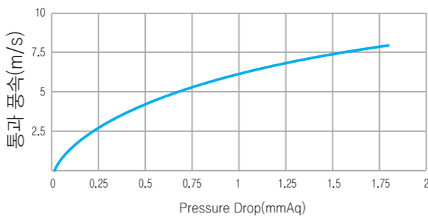
그림 9 댐퍼 압력 강하 (pressure drop of damper)
